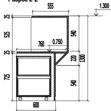
Разрез 2-2
